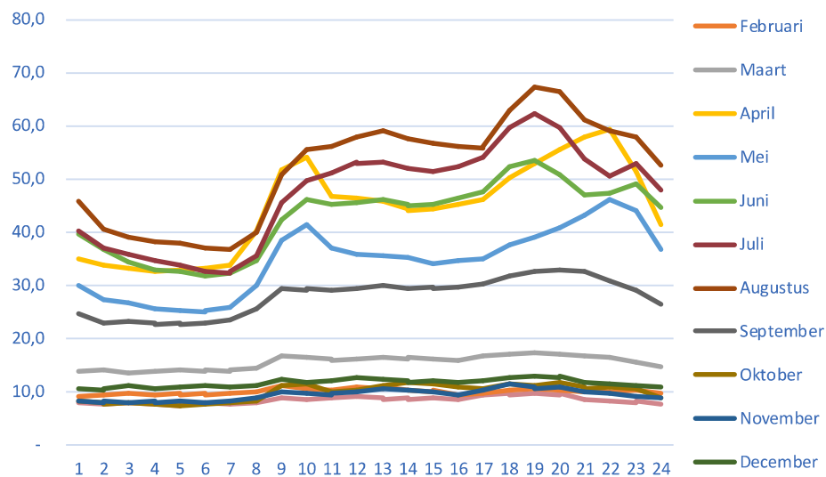
Verbruik kWh/uur, over de dag
